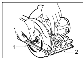
1. Llave hexagonal 2. Bloqueo del eje
